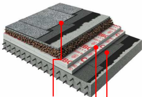
PRIMA PLAST PV - 2 lớp Xốp cách nhiệt
